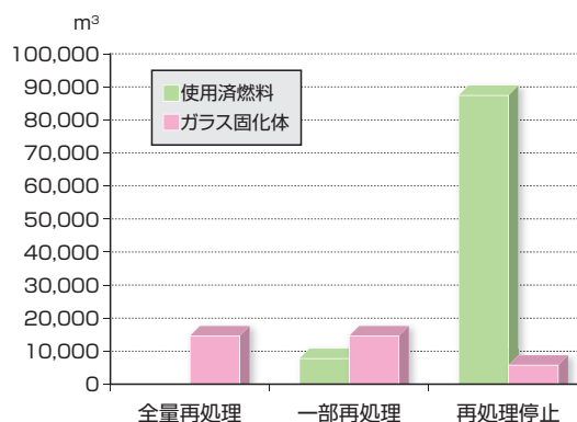
再処理シナリオ別の使用済燃料及びガラス固化体の予測発生量 (m³)
