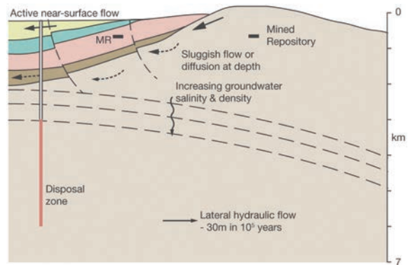
超深孔処分概念 (ブルーリボン委員会最終報告書より引用)
