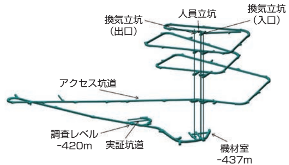
地下特性調査施設のレイアウト図
