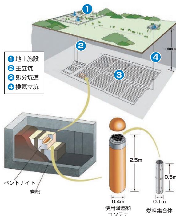
地層処分場の概念図
