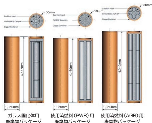
ガラス固化体と使用済燃料の処分パッケージ案
