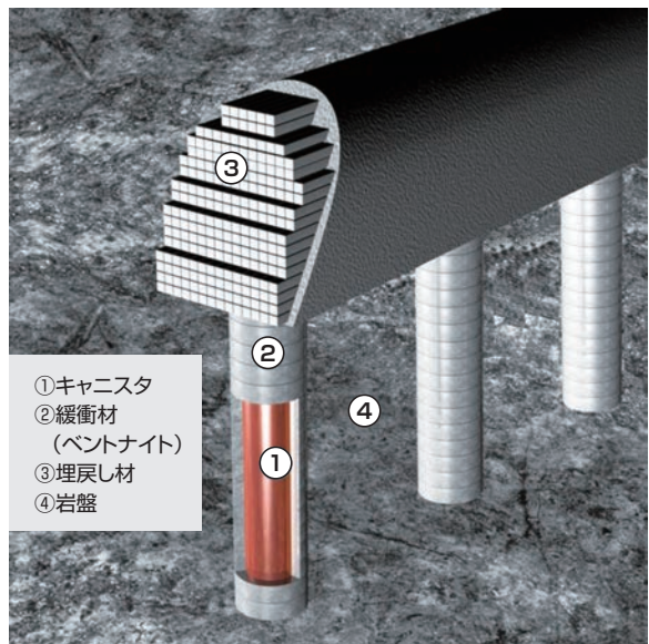
キャニスタの定置イメージ (写真提供：ポシヴァ社)
