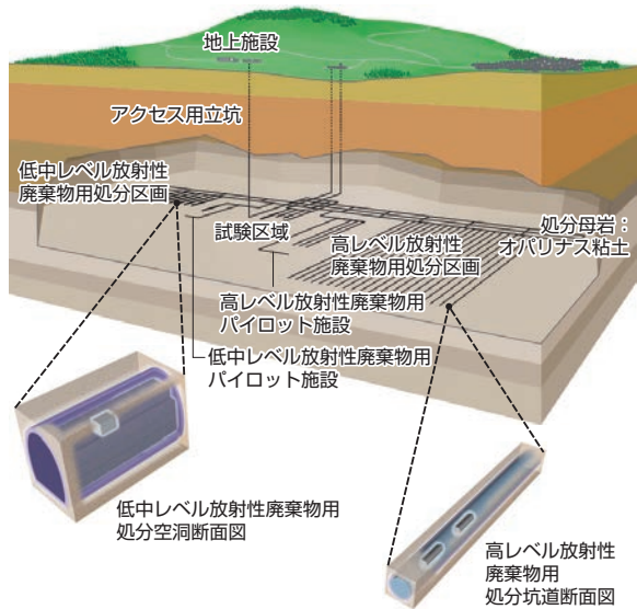
オパリナス粘土層内での複合処分場とキャニスタの定置イメージ
