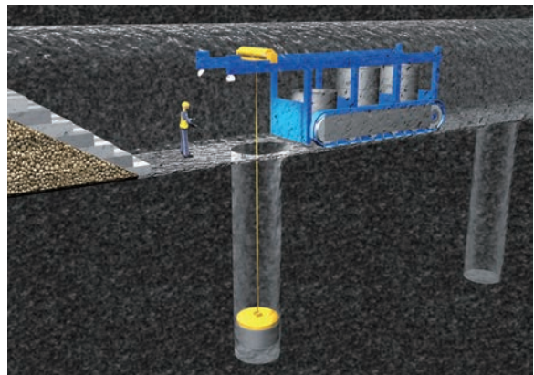
緩衝材の設置方法（概念図） (写真提供：ポシヴァ社)
