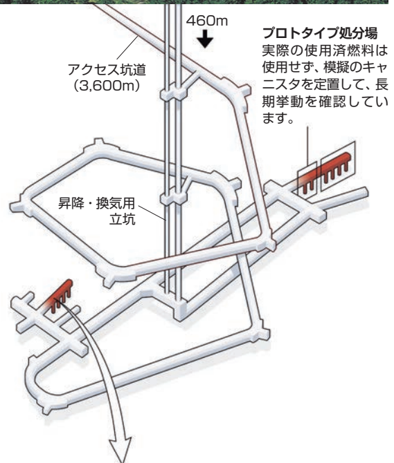
実証処分場 模擬のキャニスタを使用して装置の動作確認や作業上の問題などを確認しています。
