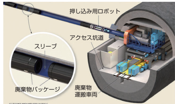
廃棄物パッケージの定置イメージ (出典：Andra)
