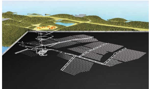
オルキルト処分場の設置イメージ (写真提供：ポシヴァ社)
