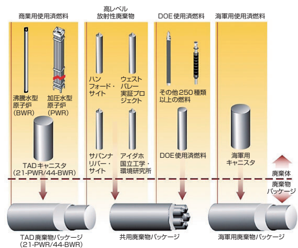
廃棄物パッケージの種類
