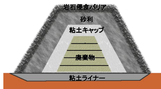
処分セルの断面イメージ図
