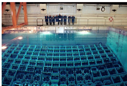
CLAB の使用済燃料の貯蔵プール
