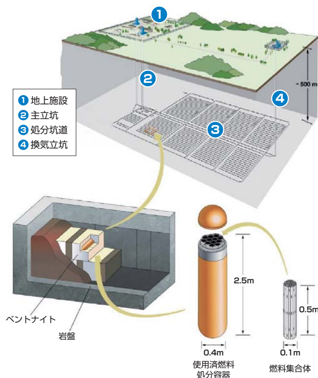
地層処分場の概念図 (出典：NWMO技術レポートTR-2017-01)
