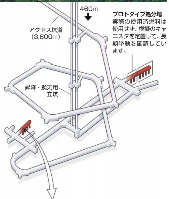
エスポ岩盤研究所の概念図 (SKB社提供資料より引用)
