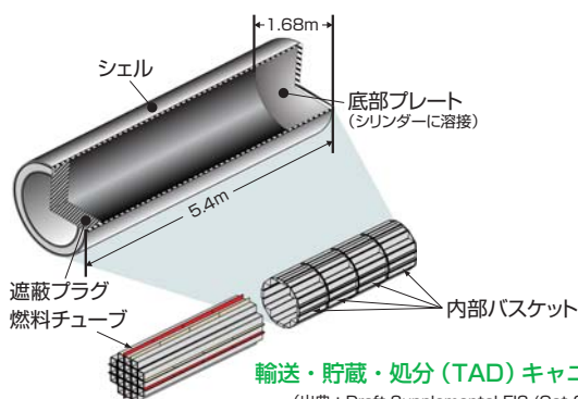
廃棄物パッケージの種類
