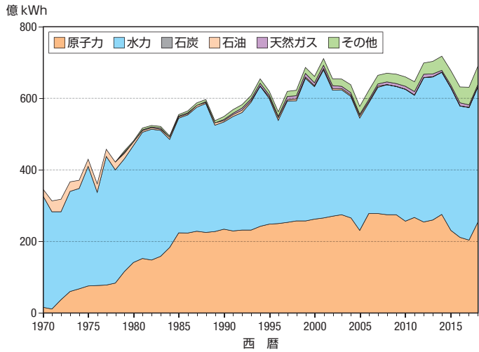
スイスの電力供給構成(発電量-2018年) (Energy Statistics 2020, IEAより作成)
