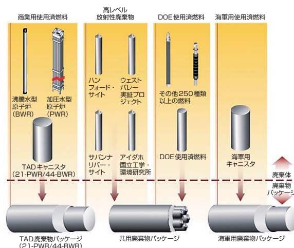
廃棄物パッケージの種類
