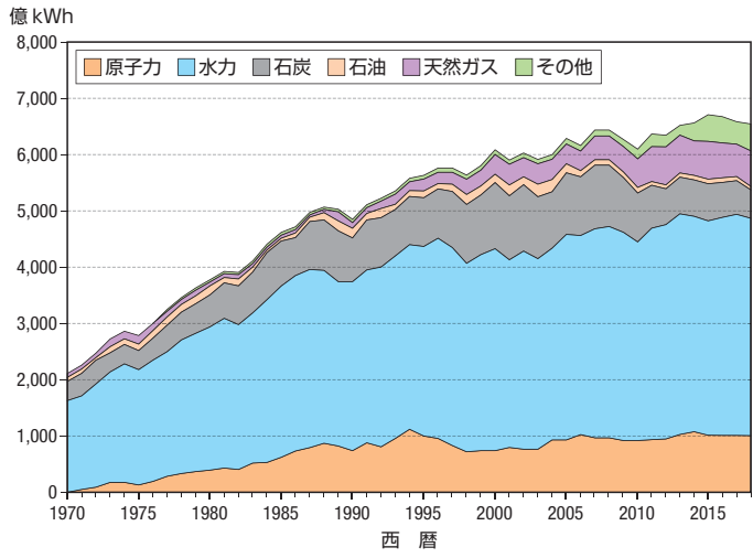
カナダの電力供給構成(発電量-2018年) (Energy Statistics 2020, IEAより作成)
