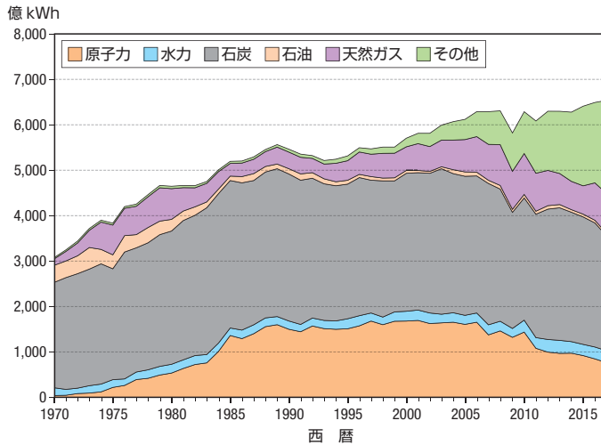
ドイツの電力供給構成(発電量-2017年) (Energy Statistics 2019, IEAより作成)
