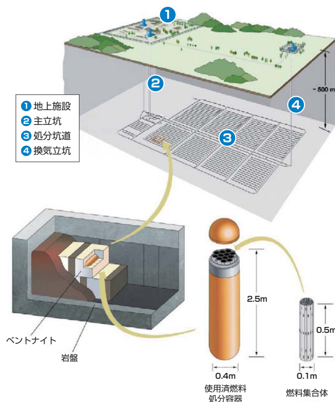
地層処分場の概念図 (出典：NWMO技術レポートTR-2018-01)
