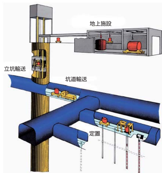
処分坑道縦置き方式
