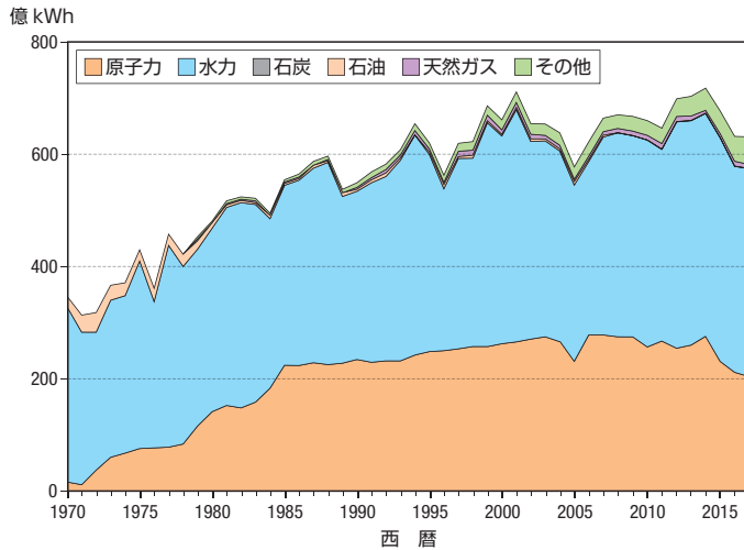
スイスの電力供給構成(発電量-2017年) (Energy Statistics 2019, IEAより作成)
