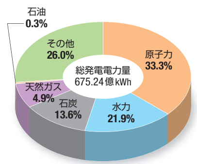
フィンランドの電力供給構成 (発電量－2017年) (Energy Statistics 2019, IEAより作成)
