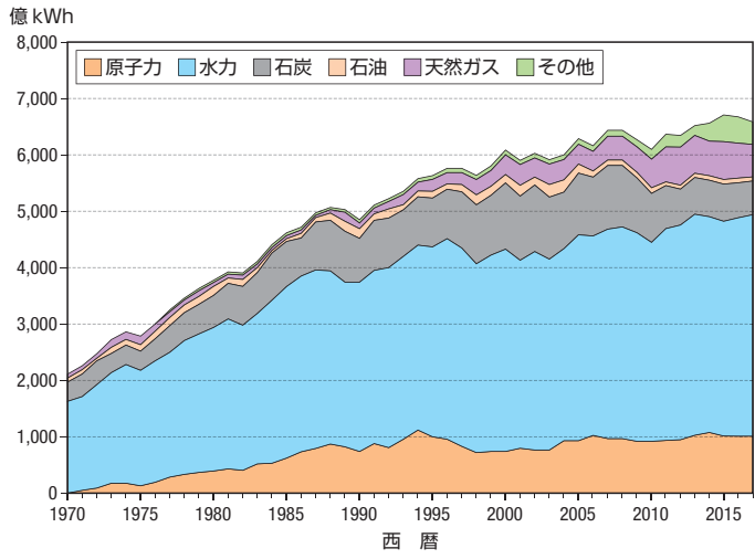
カナダの電力供給構成(発電量-2017年) (Energy Statistics 2019, IEAより作成)
