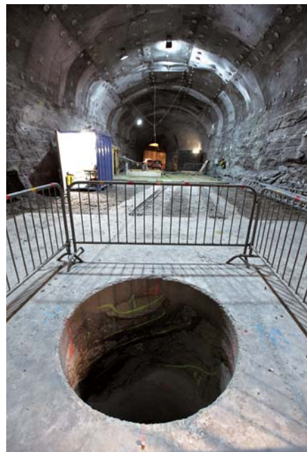
オルキルトの地下特性調査施設内の坑道と試験処分孔 （写真提供：ポシヴァ社）
